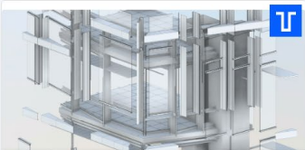
Fachada de vidrio de torre de oficinas y locales comerciales en Lima de Allende arquitectos - Modelo 3D - BIM
