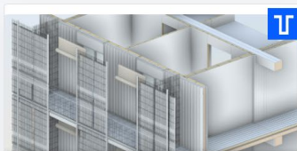
Sistema estructural en madera laminada y CLT. Viviendas sociales en Cornellà de Peris+Torral Arquitectes - Modelo 3D - BIM
